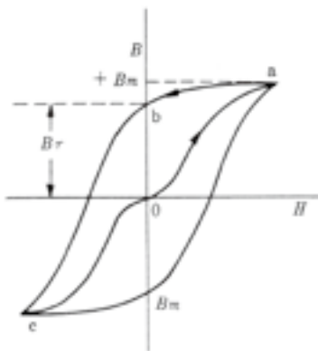
Fig. 3.4. Magnetisation curve (3)
