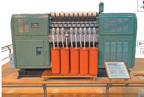
豊田ローター式オープンエンド精紡機 BD200型
